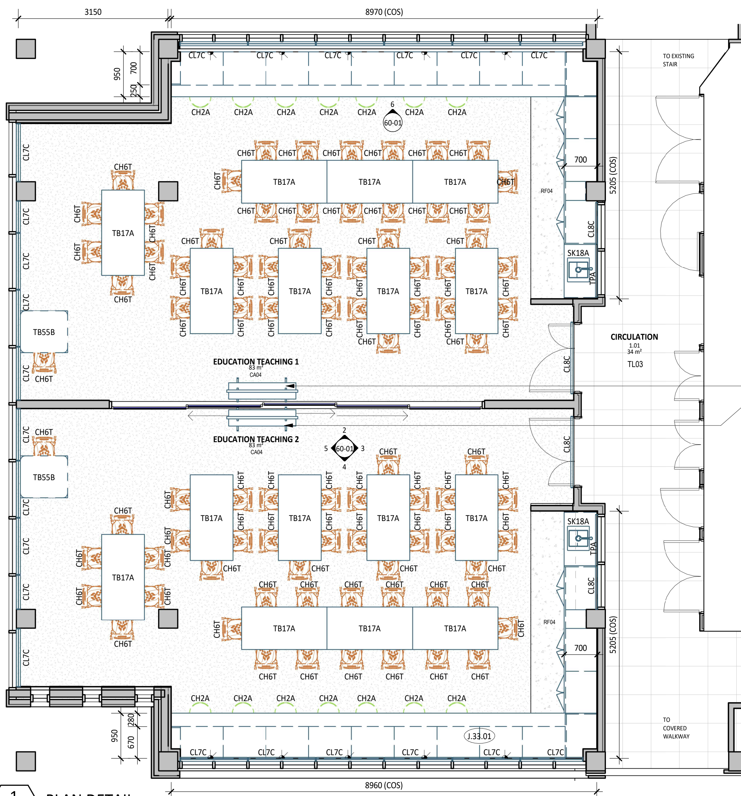
1 PLAN DETAIL 1 : 50
